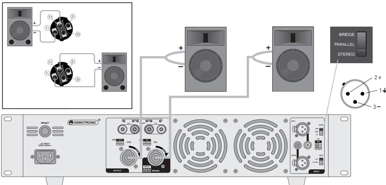
Abb. 1 Verwendung der Speaker-Buchsen im Stereobetrieb
