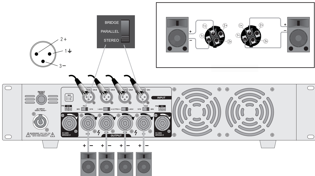
Abb. 7 Verkabelung im Stereobetrieb
